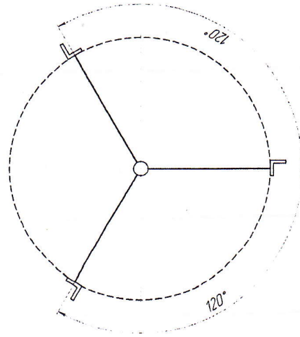
Рисунок 1 – Схема размещения растяжек в плане
